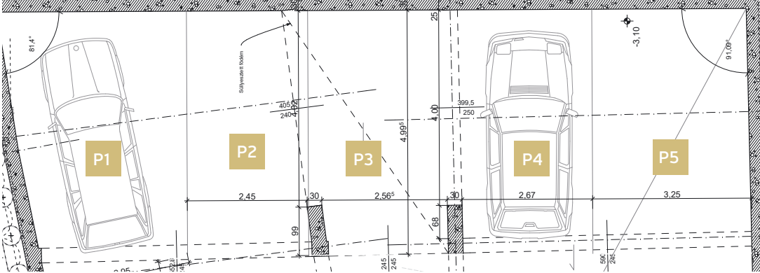
Normál Parkoló | Mélygarázs | C épület | P1-5
